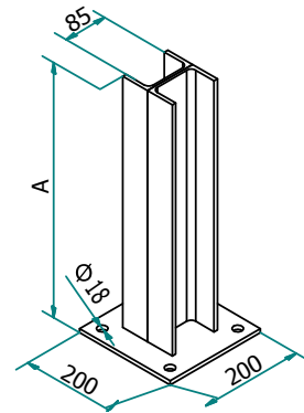
Profilé double PB-D
