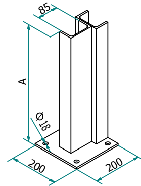
Profilé double PB-90°
