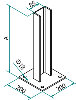
Profilé simple PB-S
