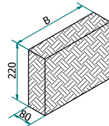
Poutre Bois PB
