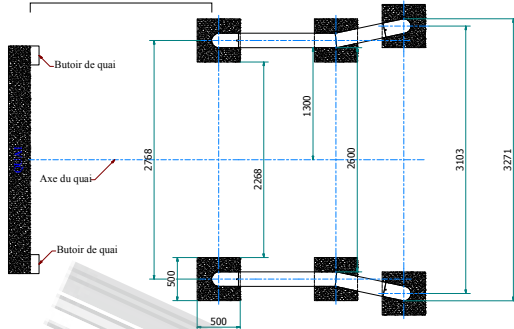
Schéma d'installation du Q20-1071
