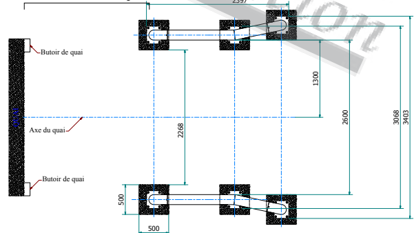
Schéma d'installation du Q20-1070
