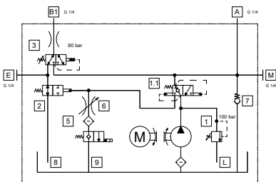
T20-0001 Groupe hydraulique 1 électrovanne 24 VAC 50 Hz pour mini-rampe type MRBH/PAF-H
