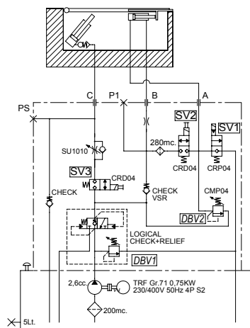
T30-0026 Groupe hydraulique 3 électrovanne 24 VDC pour niveleur à lèvre télescopique
