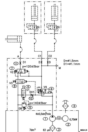
T30-3047 Groupe hydraulique 1 électrovanne 24 VDC pour niveleur à barette rabattable
