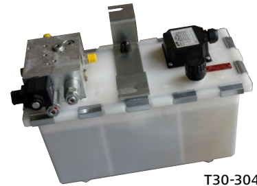
T30-3047 Groupe hydraulique 1 électrovanne 24 VDC pour niveleur à barette rabattable
