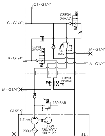
T30-00027 Groupe hydraulique 3 électrovanne 24 VAC 50 Hz pour niveleur à lèvre télescopique
