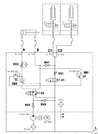
T30-3041 Groupe hydraulique 2 électrovanne 24 VDC pour niveleur à lèvre télescopique
