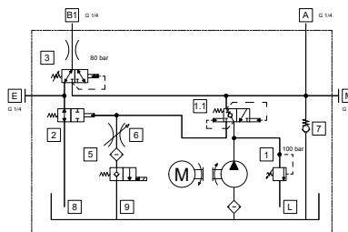
T30-3035 Groupe hydraulique 1 électrovanne 24 VAC 50 Hz pour niveleur à barette rabattable
